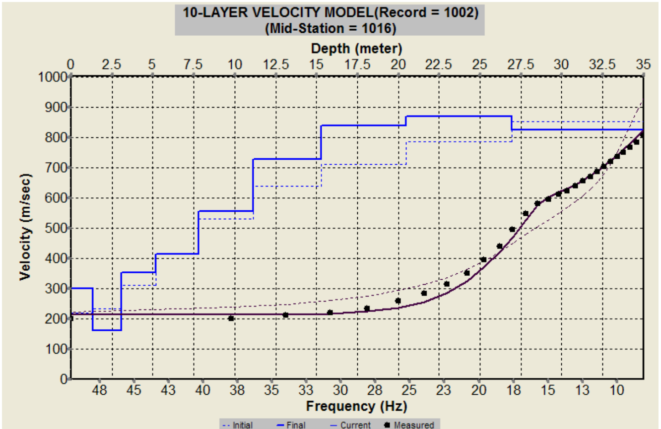
Fig. 48 – Profilo verticale 1D delle V_S ottenuto dall’inversione della curva di dispersione della velocità di fase delle onde superficiali di Rayleigh: MASW n. 4 - acquisizione n. 2.
