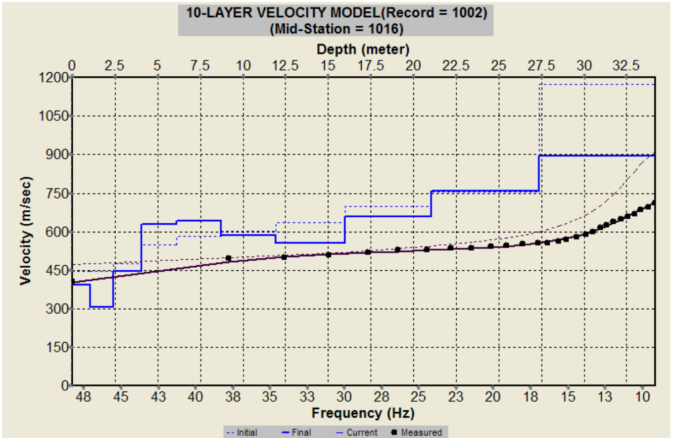
Fig. 34 – Profilo verticale 1D delle V_S ottenuto dall’inversione della curva di dispersione della velocità di fase delle onde superficiali di Rayleigh: MASW n. 2 - acquisizione n. 2.
