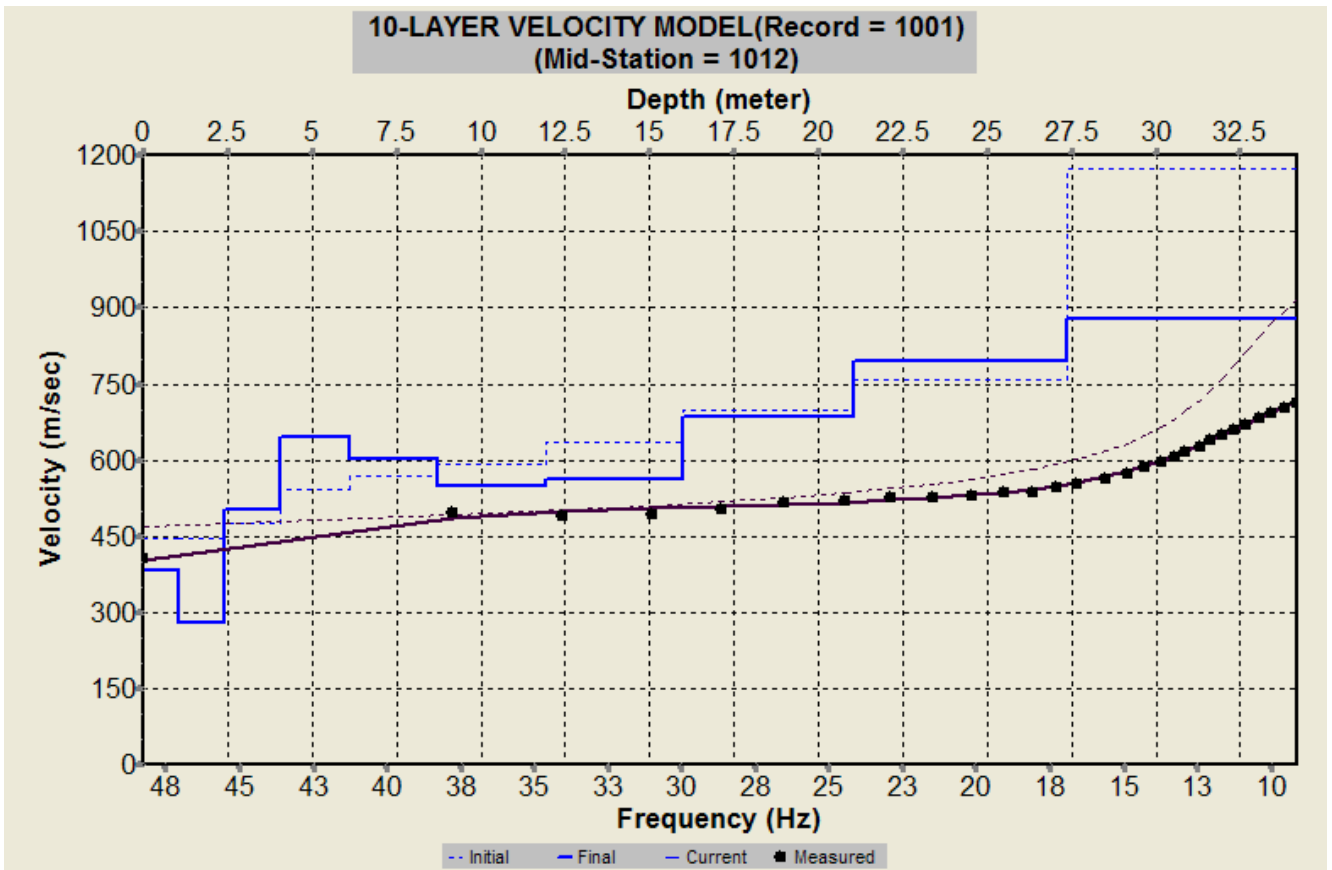
Fig. 33 – Profilo verticale 1D delle V_S ottenuto dall’inversione della curva di dispersione della velocità di fase delle onde superficiali di Rayleigh: MASW n. 2 - acquisizione n. 1.
