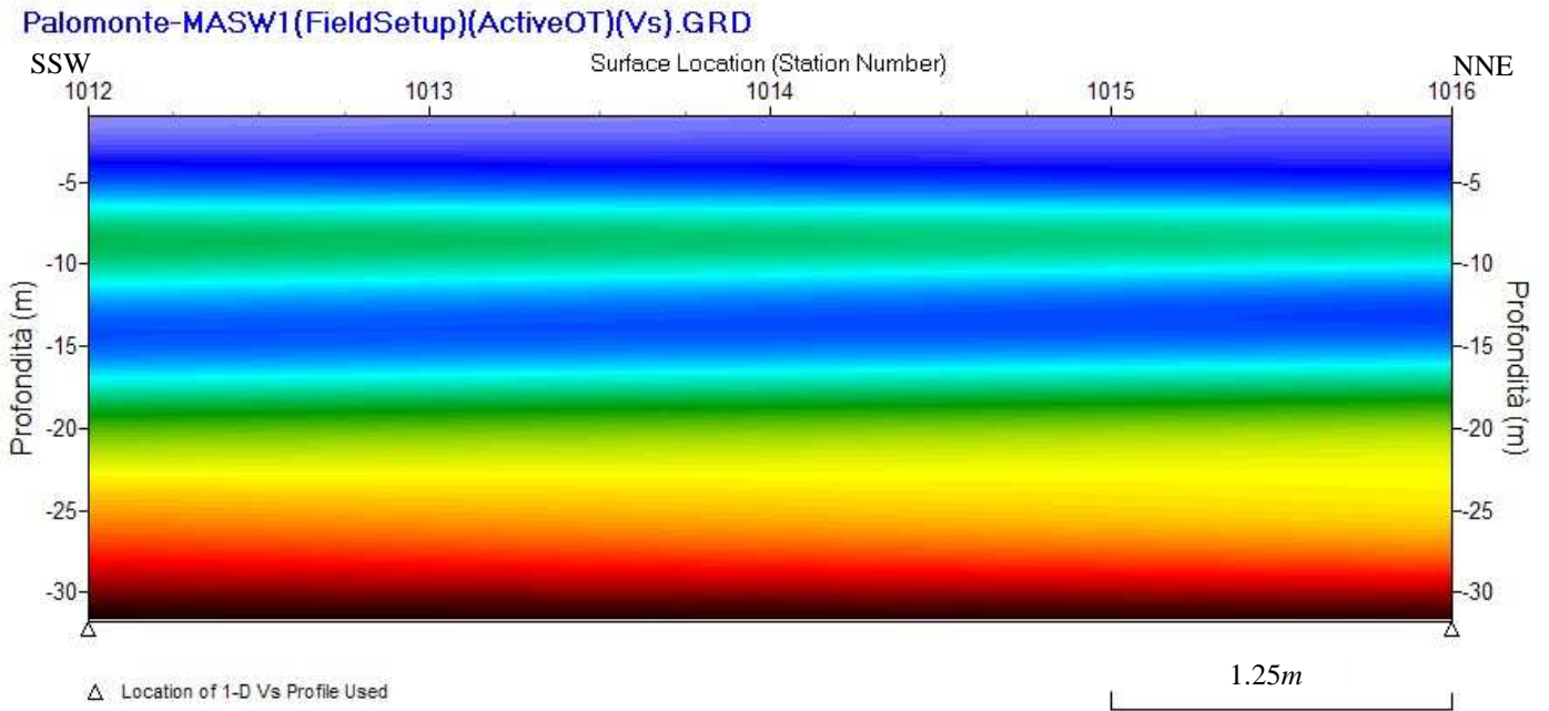
Fig. 28 – Modello sismostratigrafico 2D delle V_s ottenuto dall'indagine Sismica MASW n. 1.
