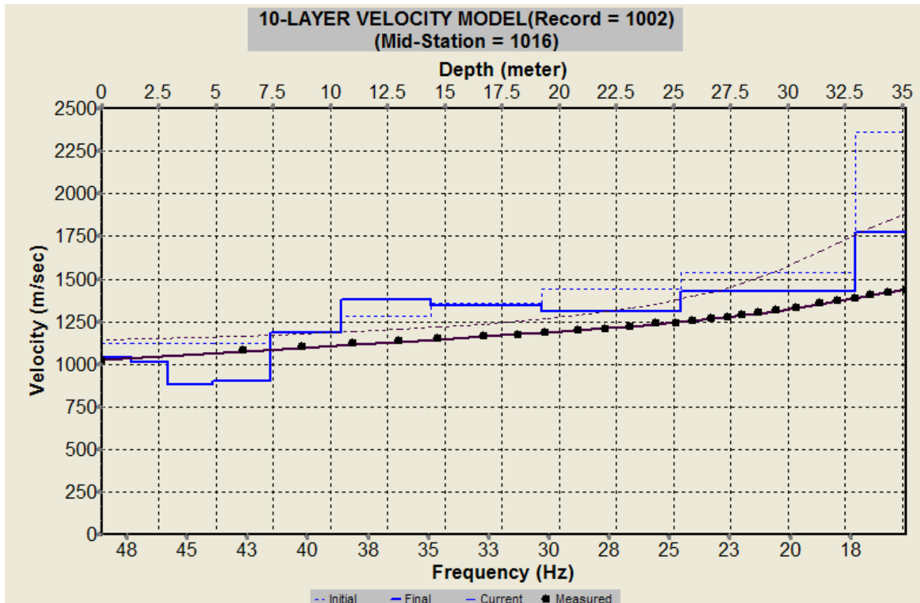
Fig. 62 – Profilo verticale 1D delle V_s ottenuto dall’inversione della curva di dispersione della velocità di fase delle onde superficiali di Rayleigh: MASW n. 6 - acquisizione n. 2.
