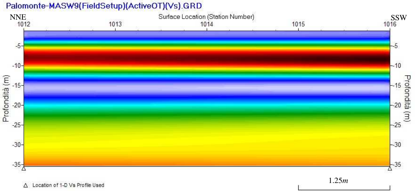
Fig. 84 – Modello sismostratigrafico 2D delle V_s ottenuto dall'indagine Sismica MASW n. 9.
