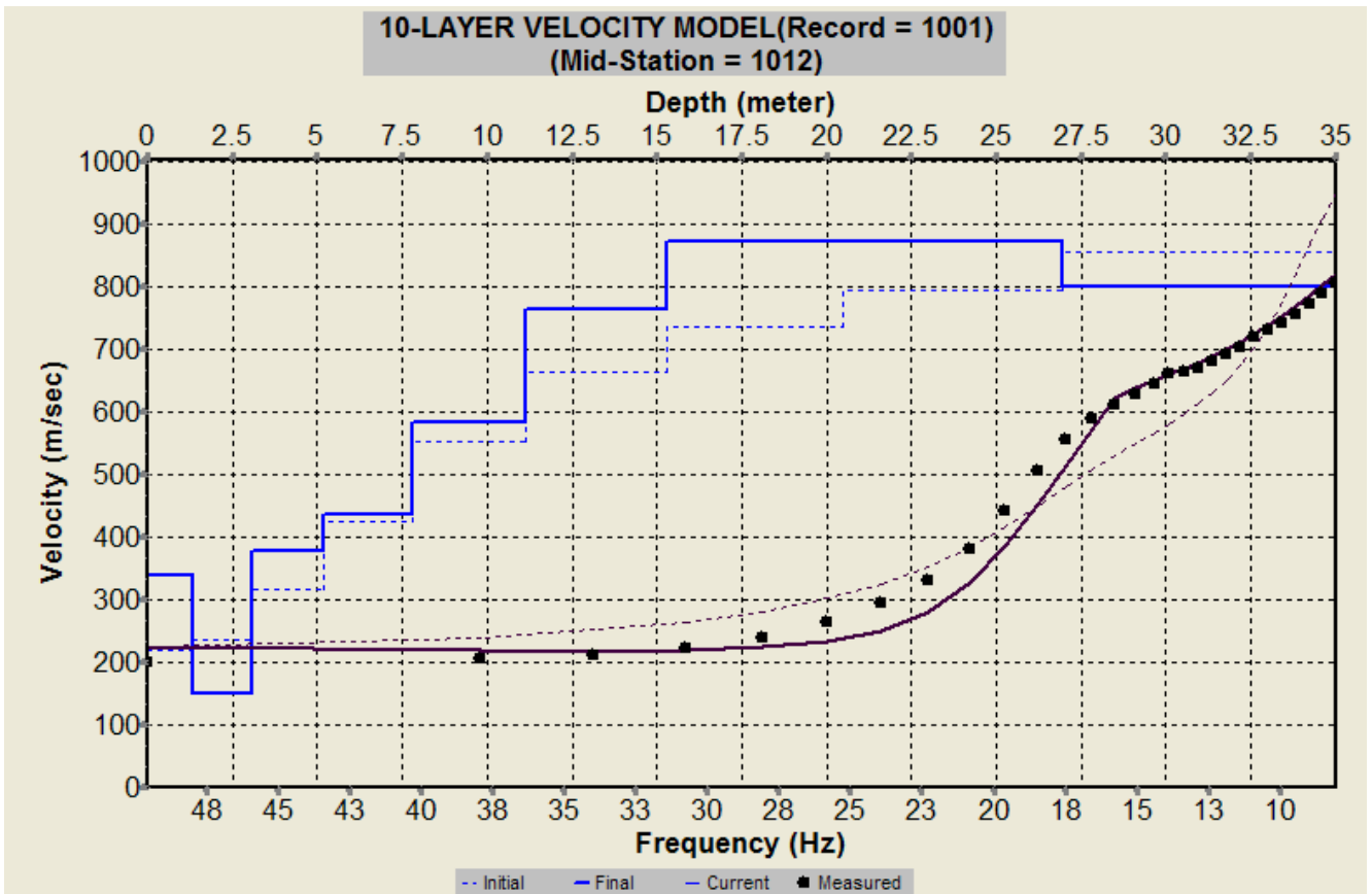
Fig. 47 – Profilo verticale 1D delle V_S ottenuto dall’inversione della curva di dispersione della velocità di fase delle onde superficiali di Rayleigh: MASW n. 4 - acquisizione n. 1.
