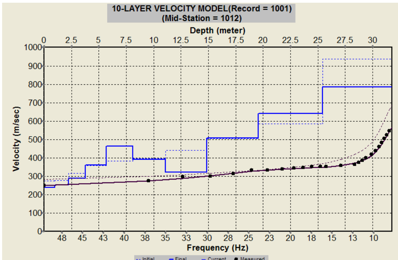
Fig. 26– Profilo verticale 1D delle V_S ottenuto dall’inversione della curva di dispersione della velocità di fase delle onde superficiali di Rayleigh: MASW n. 1 - acquisizione n. 1.
