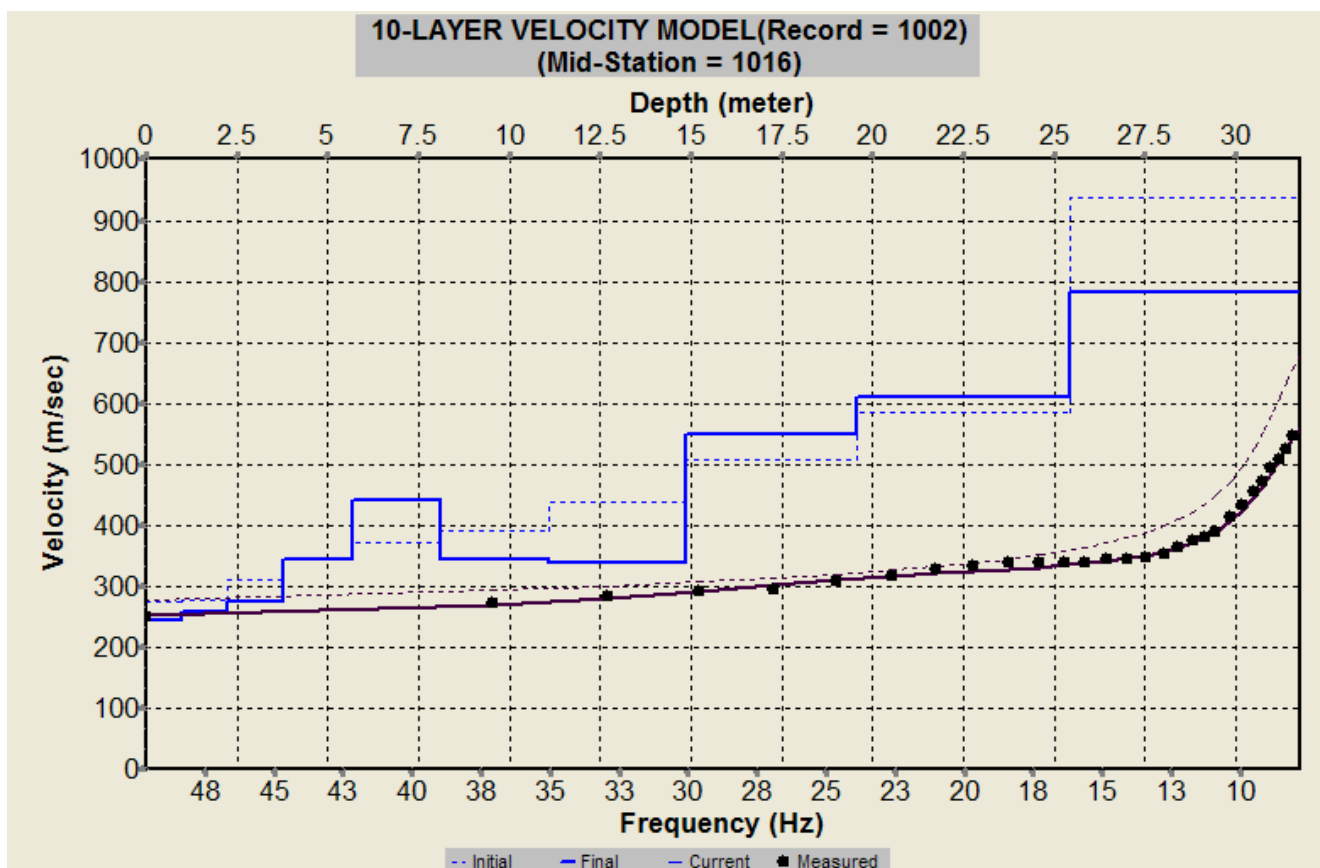
Fig. 27 – Profilo verticale 1D delle V_S ottenuto dall’inversione della curva di dispersione della velocità di fase delle onde superficiali di Rayleigh: MASW n. 1 - acquisizione n. 2.
